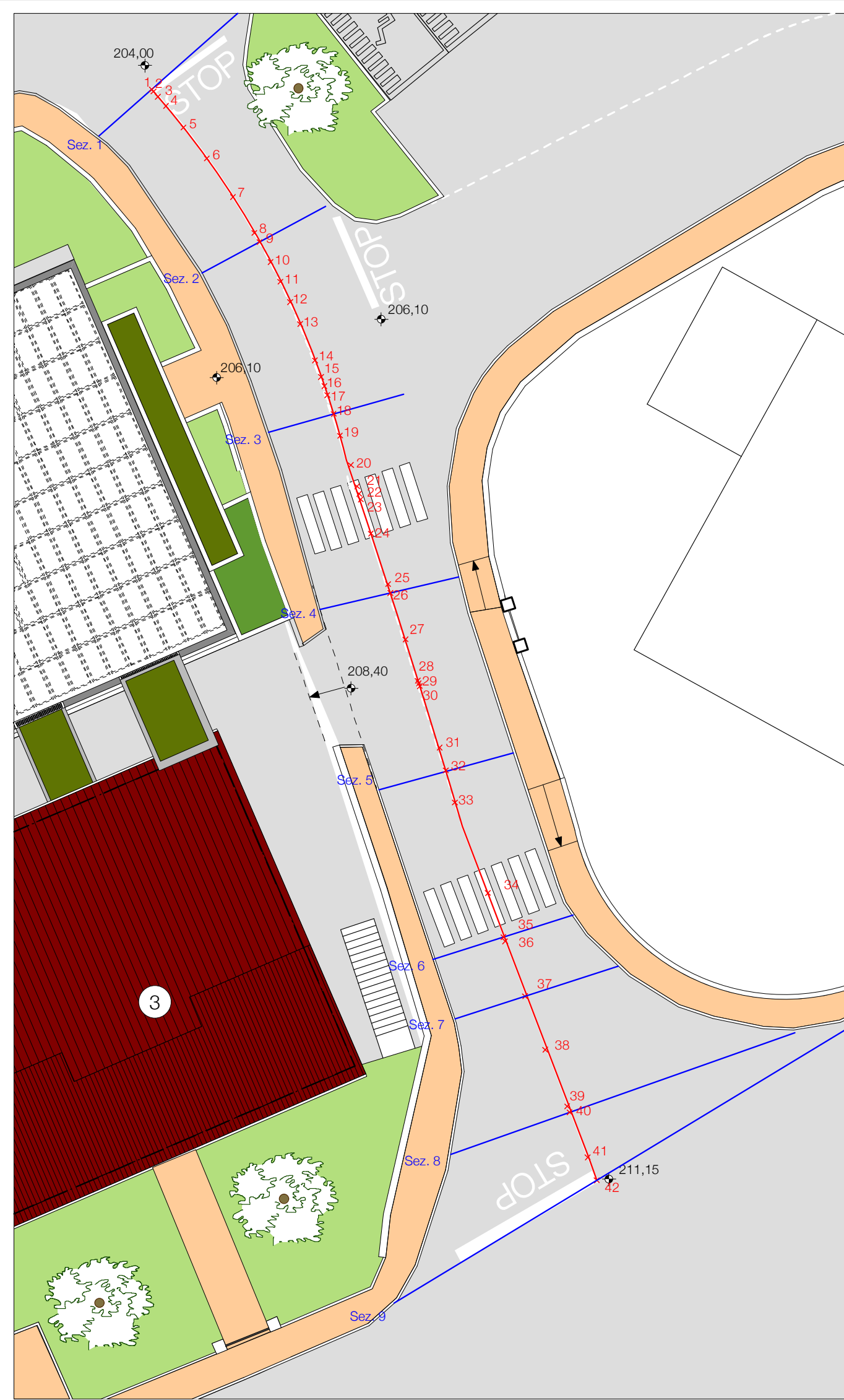
Planimetria tratto stradale (rap. 1:200)
