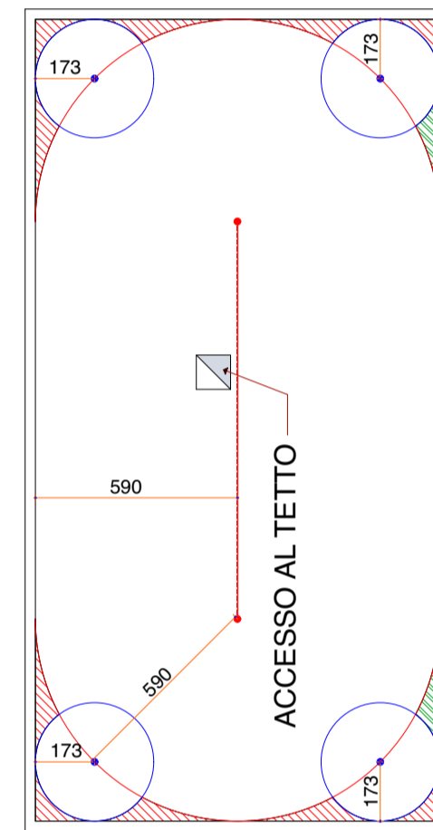
PIANTA DELLA COPERTURA EDIFICIO S
