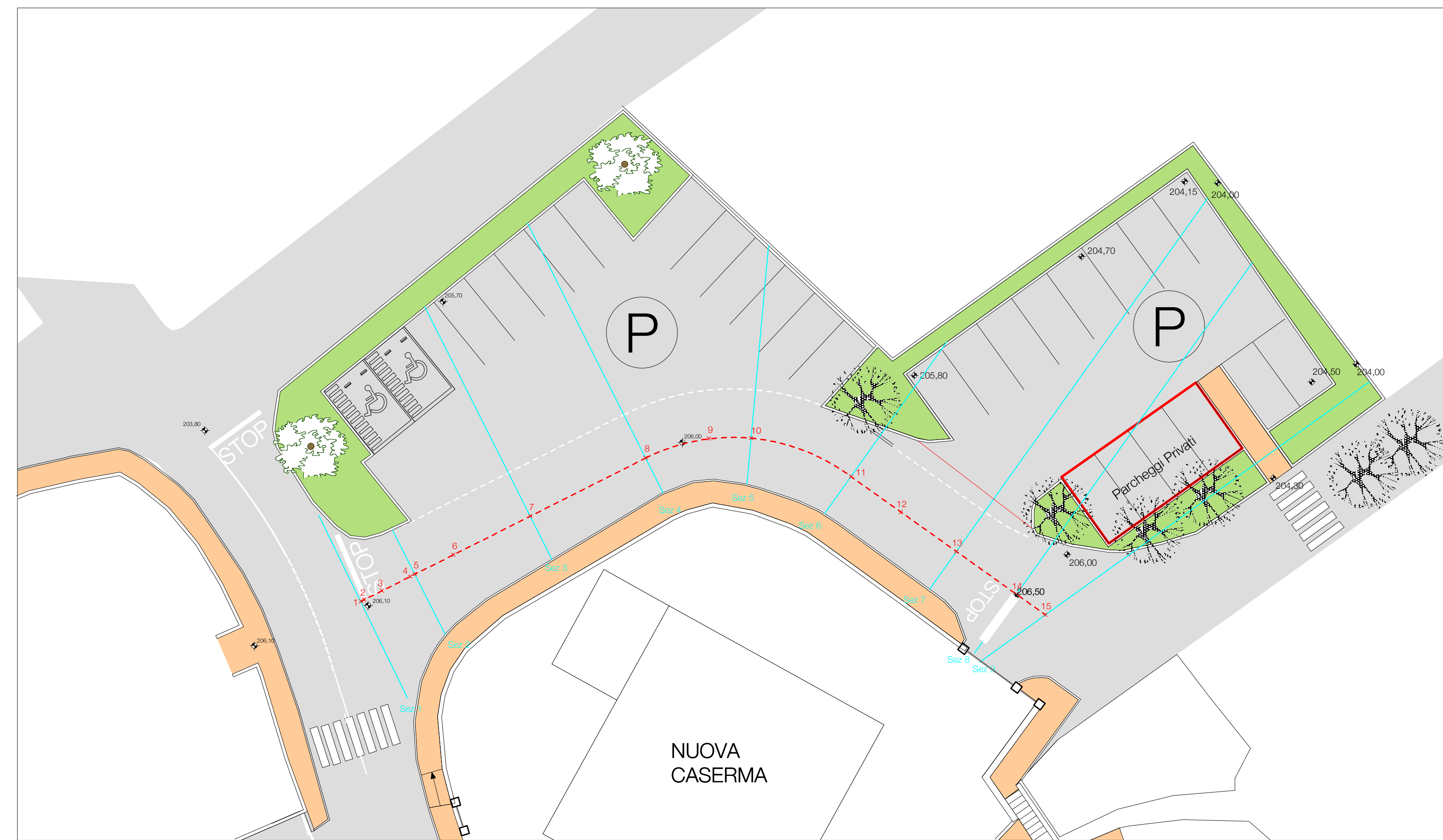
Planimetria tratto stradale (rapp. 1:200)
