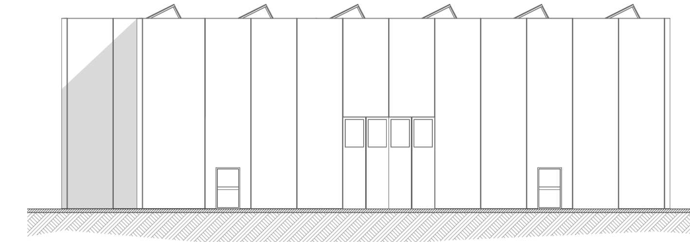
PROSPETTO SUD - EST
