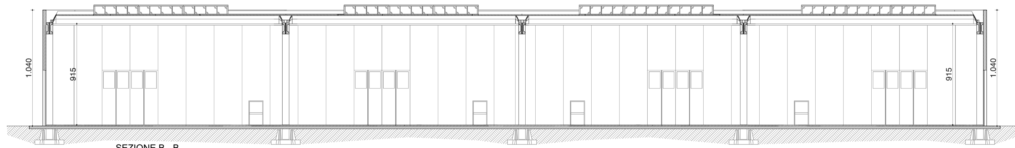
SEZIONE B - B
